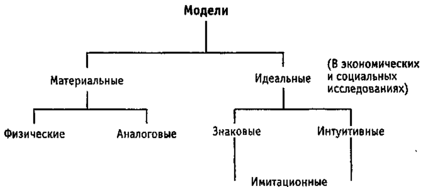
Рис. 2. Классификация моделей
